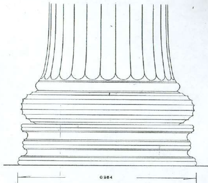
Εἰκ. 1. Βάση ἰωνικοῦ κίονα τοῦ ναοῦ τῆς Θέρμης. (Σχέδιο Ι. Τραυλοῦ).
